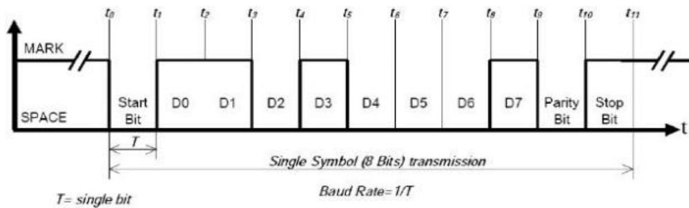
图 4-6 UART 数据字节格式
